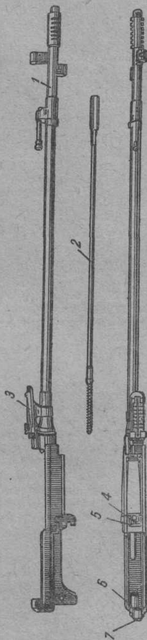
Фиг. 440. Ствол со ствольной коробкой.
