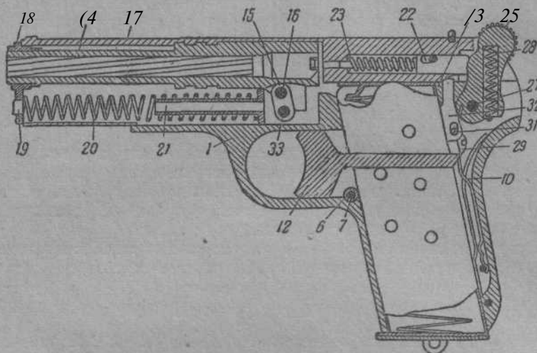
Фиг. 237. Разрез пистолета по оси.
