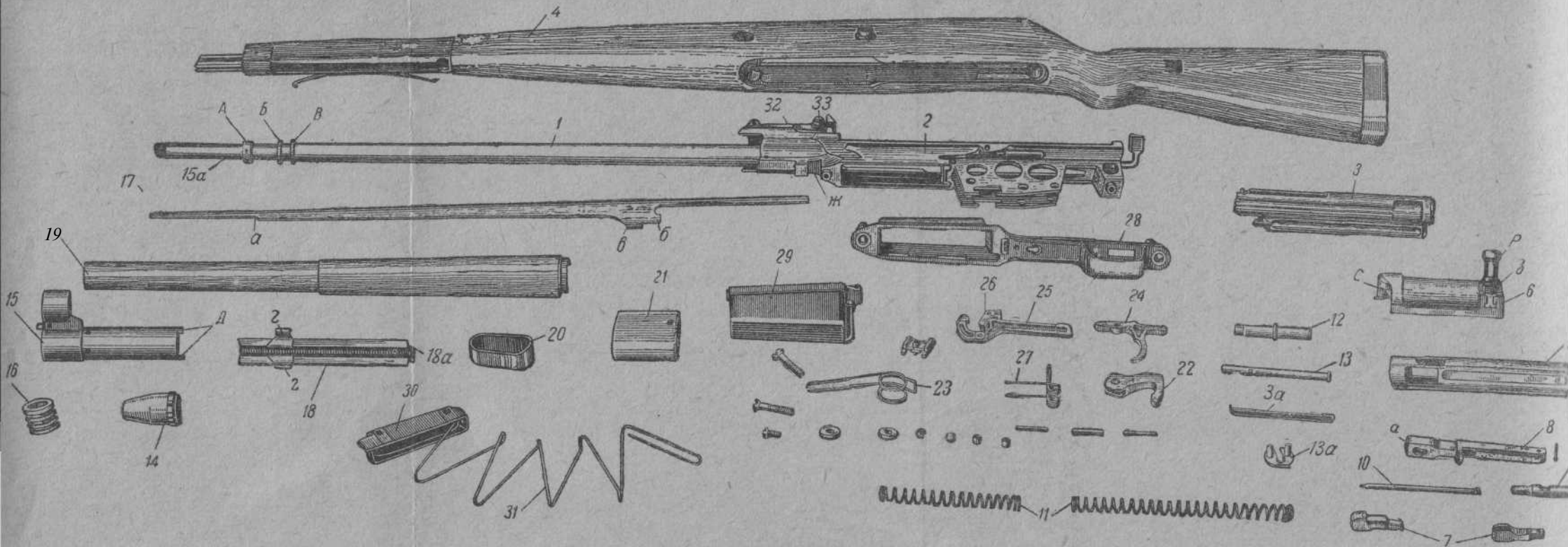
Фиг. 557. Детали германской самозарядной винтовки 0-41 (W).
