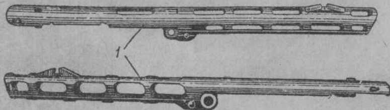
Фиг. 364. Ствольная коробка.
