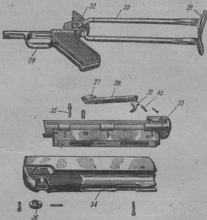
Фиг. 400. Приклад разобранный.
