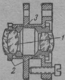
Фиг. 460. Разрез обора- рачивающей системы.
