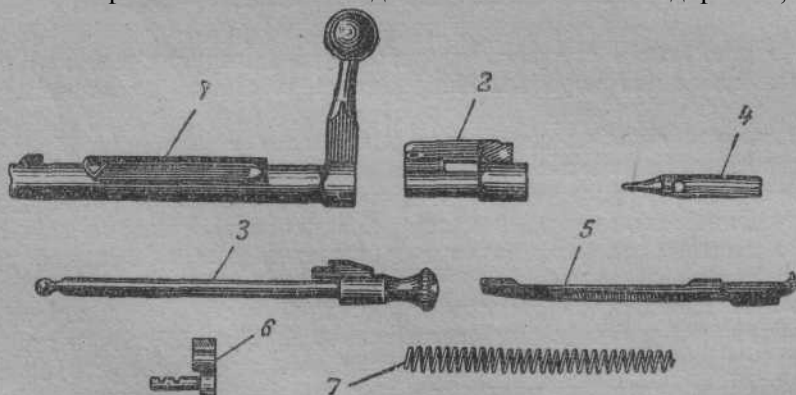
Фиг. 181. Детали затвора:
