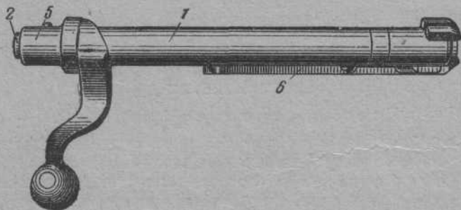
Фиг. 149. Затвор (собранный).
