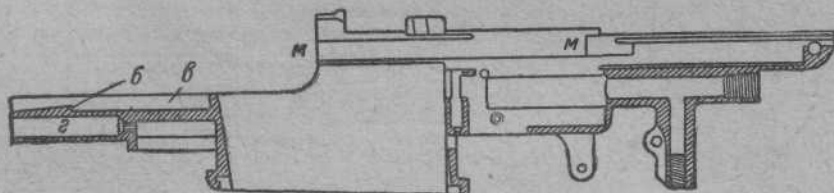
Фиг. 474. Коробка в разрезе.
