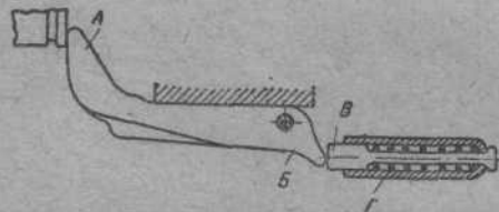
Фиг. 563. Отражатель.
