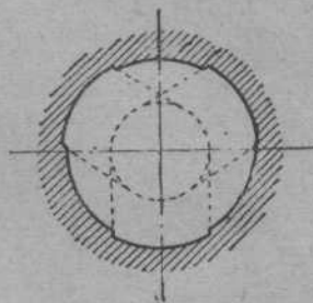
Фиг. 74. Нарезы 7,5-лш винтовки системы Шмидт-Рубина обр. 1889/1896 гг.
