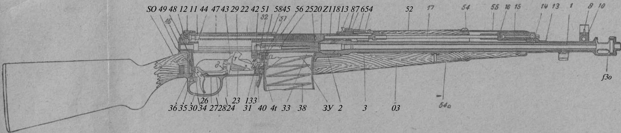
Фиг. 446. Разрез карабина Токарева.
