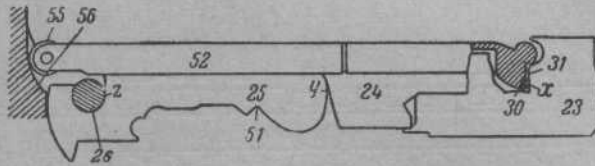
Фиг. 501. Затвор.
