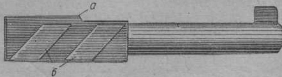
Фиг. 333. Ствол.
