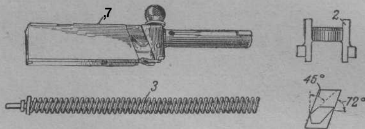
Фиг. 414. Затвор с возвратной пружиной.
