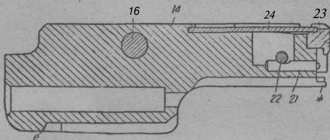
Фиг. 369. Затвор.
