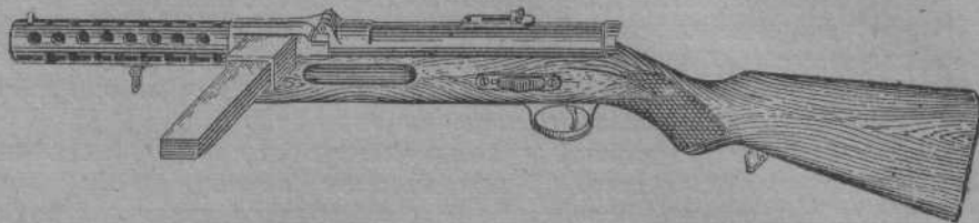
Фиг. 381. Пистолет-пулемет Рейнметалл обр. 1920 г. (вид слева).
