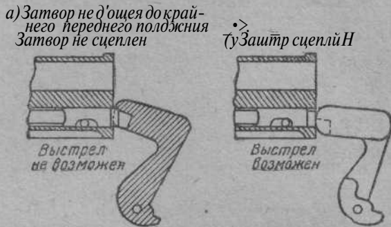
Фиг. 485. Предохранитель от преждевременных выстрелов.
