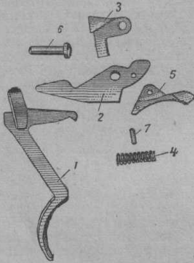
Фиг. 191. Спусковой механизм.
