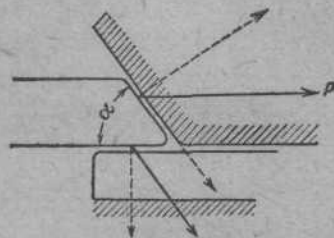
Фиг. 545б. Действие сил при выстреле.
