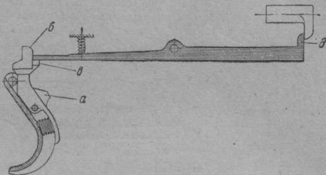
Фиг. 315. Схема работы спускового механизма.
