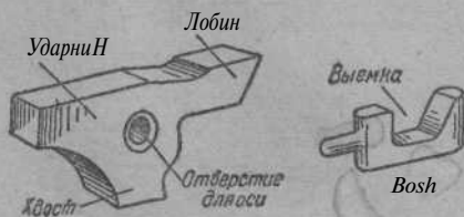
Фиг. 350. Ударник и боек.
