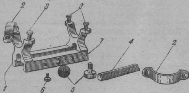
Фиг. 122. Кронштейн.
