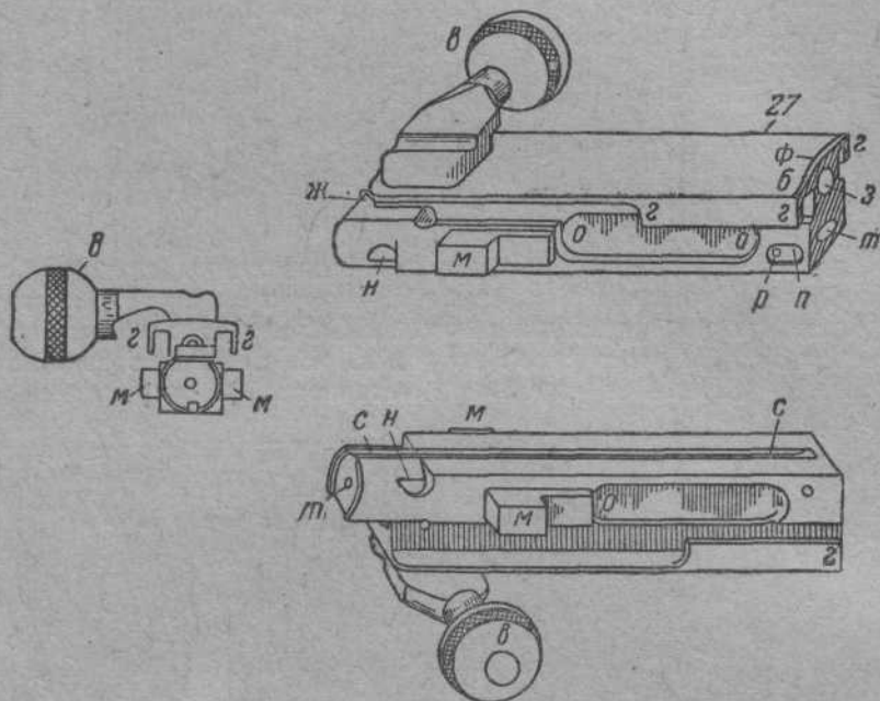
Фиг. 476. Затвор.
