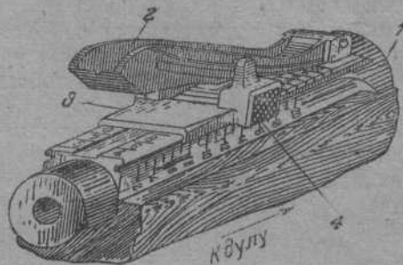
Фиг. 136. Секторный прицел.
