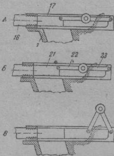
Фиг. 81. Схема работы механизма
