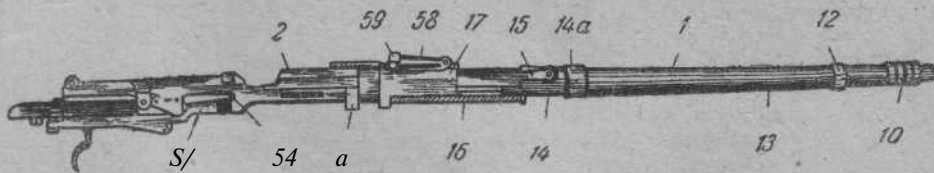
Фиг 552. Ствол с коробкой.
