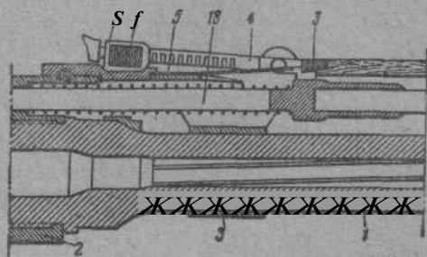
Фиг. 442. Прицельное пришоообление.
