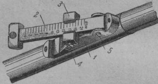
Фиг. 185. Прицел.
