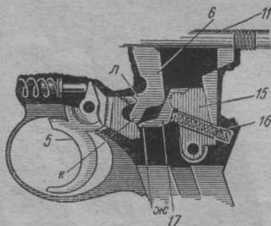
Фиг. 302. Схема работы ударно-спускового механизма
