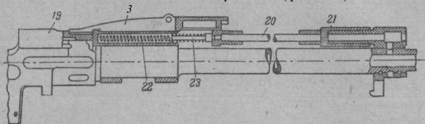
Фиг. 427. Механизм отпирания.
