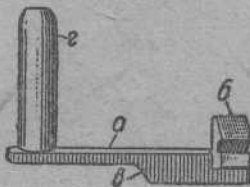
Фиг. 262. Затворная задержка.
